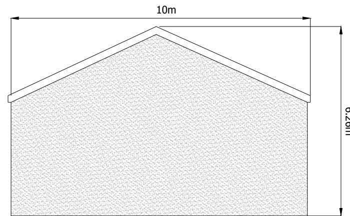
END ELEVATION
